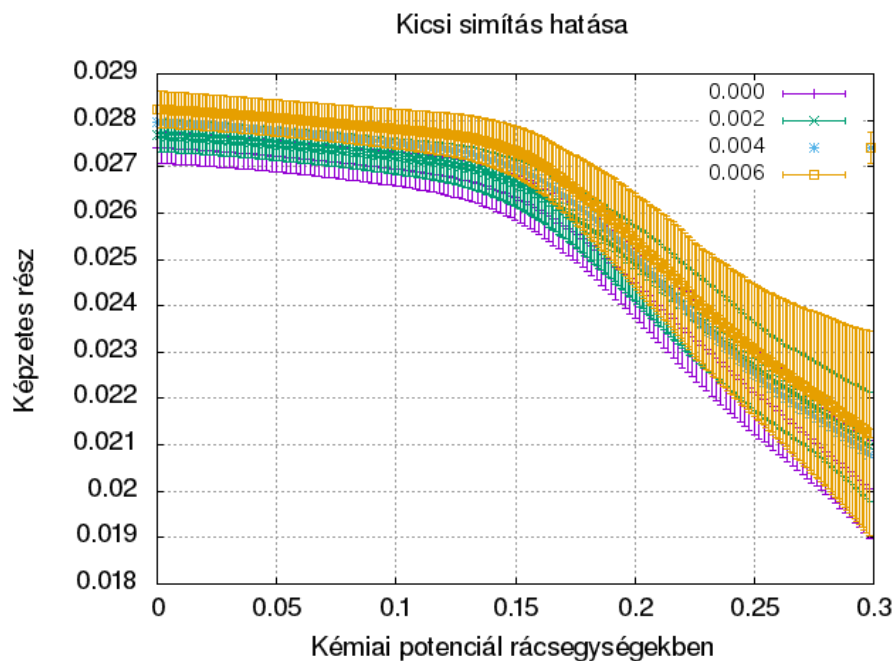
9. ábra. Kis simítás hatása a képzetes részekre, amik is simítás értékek esetén alig mozdulnak el.
