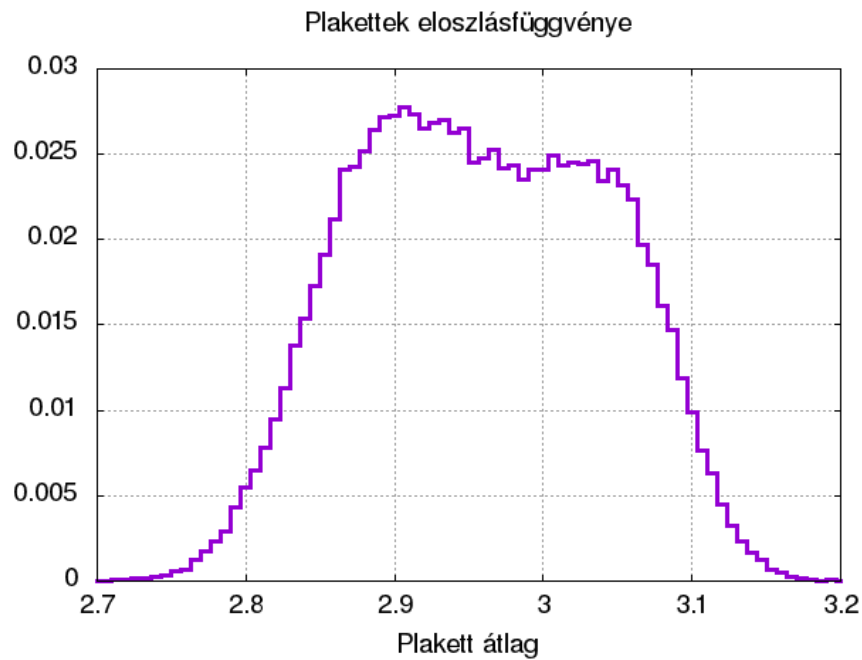
3. ábra. Plakettek eloszlása N_s=6 -os rács esetén, ahol \beta = 5.188 . Jól látható a kettős csúcs, amely a két fázis jelenlétét jelzi
