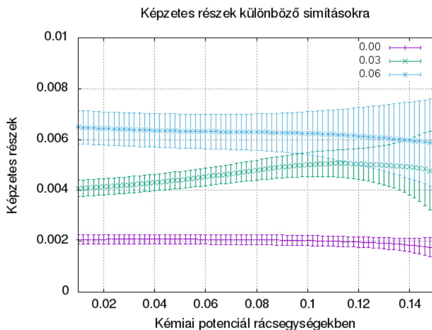
14. ábra. Végtelen térfogati extrapolált képzetes részek különböző simításokra
