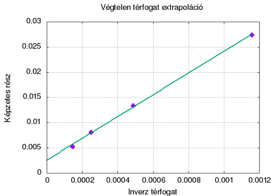
5. ábra. Végtelen térfogati extrapoláció zérus kémiai potenciál esetén. Végess helyen metszi a tengelyt az egyenes, ami analitikus átmenetre utal.
